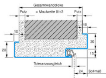
Umfassungszarge (UZS) Profil 23
