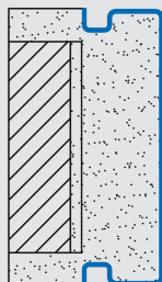
Durchgangszarge mit Schattennut
