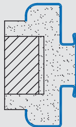
Doppeltürzarge mit Radius
