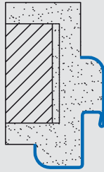
Eckzarge mit Radius
