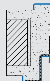
Umfassungszarge mit Bleieinlage (Strahlenschutz)
