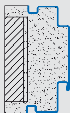
Zierfalz zarge mit Schattennut
