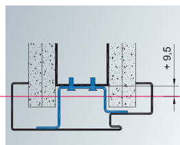
Standard-Zargen für Ständerwerk, Profil 23/1645
