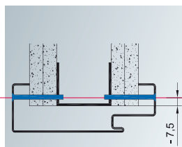
3-teilige Steckzarge, Profil 23/1645
