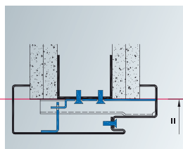
2-teilig in Nut verschraubt, Profil 2140/1645
