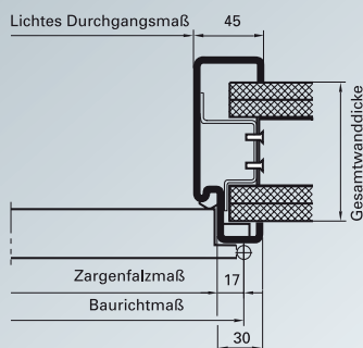
Horizontaler Schnitt Zarge mit Wand Ständerwerk
