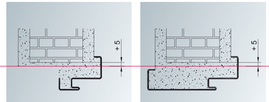
Standard-Zargen für Mauerwerk, Gipswand und Ytong-Stein
