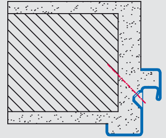
Eckzarge mit Dübelstanzung im Nutbereich (Sanierung)
