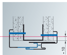
2-teilig mit Trennfuge, Profil 2150/0045
