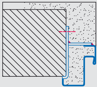
Eckzarge mit Dübellochstanzung im Nutbereich (Sanierung)
