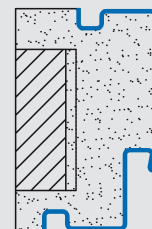
Umfassungszarge mit Schattennut
