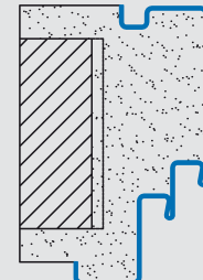
Doppelfalz zarge mit 1-seitiger Schattennut
