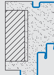
Doppelfal zarge mit 1-seitiger Schattennut
