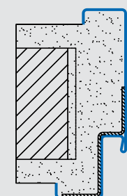
Umfassungszarge mit Bleieinlage (Strahlenschutz)
