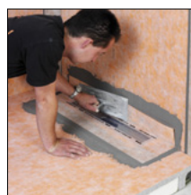
zu 4. KERDI-Manschette mit KERDI-COLL aufkleben
