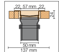
Querschnitt Miteleinbau
