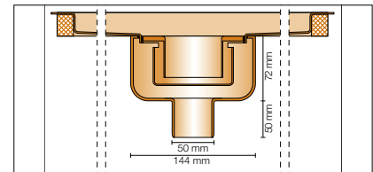
Längsschnitt Wand- /Miteleinbau
