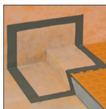
Bei Bedarf stehen passende Formteile Schlüter®-KERDI-KERS für die Gefälleabdichtung zur Verfügung
