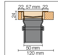
Querschnitt Wandeinbau
